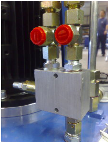
Tryckbegränsningsventil
